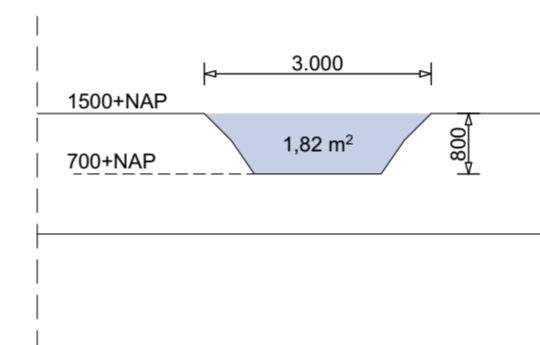
Doorsnede A-A nieuwe sloot middendoor
