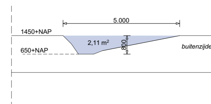
Doorsnede C-C nieuwe sloot rondom
