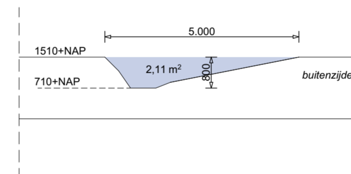
Doorsnede B-B nieuwe sloot rondom
