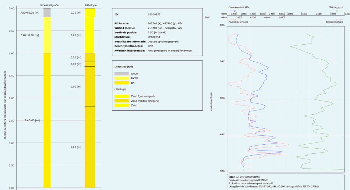
Figuur 2 Bodemopbouw (links) en conusweerstand, indicatie van hoe stijf de grond is (rechts).
